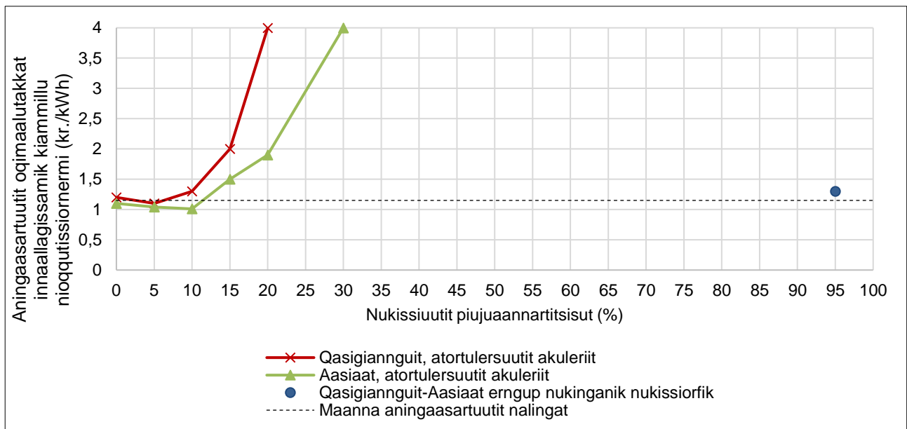
Figuri 4. Nukimmik nioqutissiornermi aningaasartuutit piujuaannartitsisumik nukissiuuteqarnermut sanilliullugu
