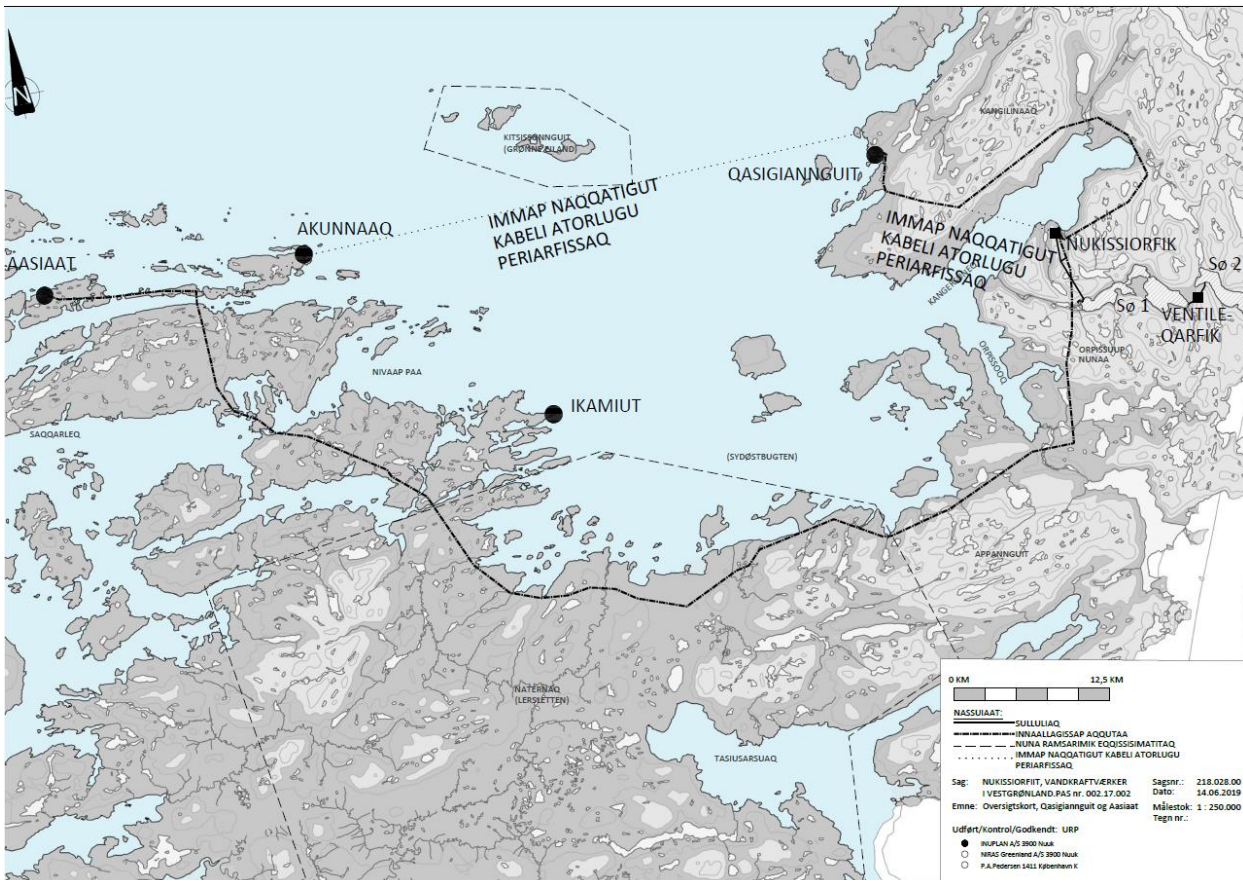
Figuri 3. Qasigiannuguit aamma Aasiaat erngup nukinganik iluaquteqarluni nukissiorfimmiit pilersorneqalernissaannut nunap assinga takussutissiisoq
