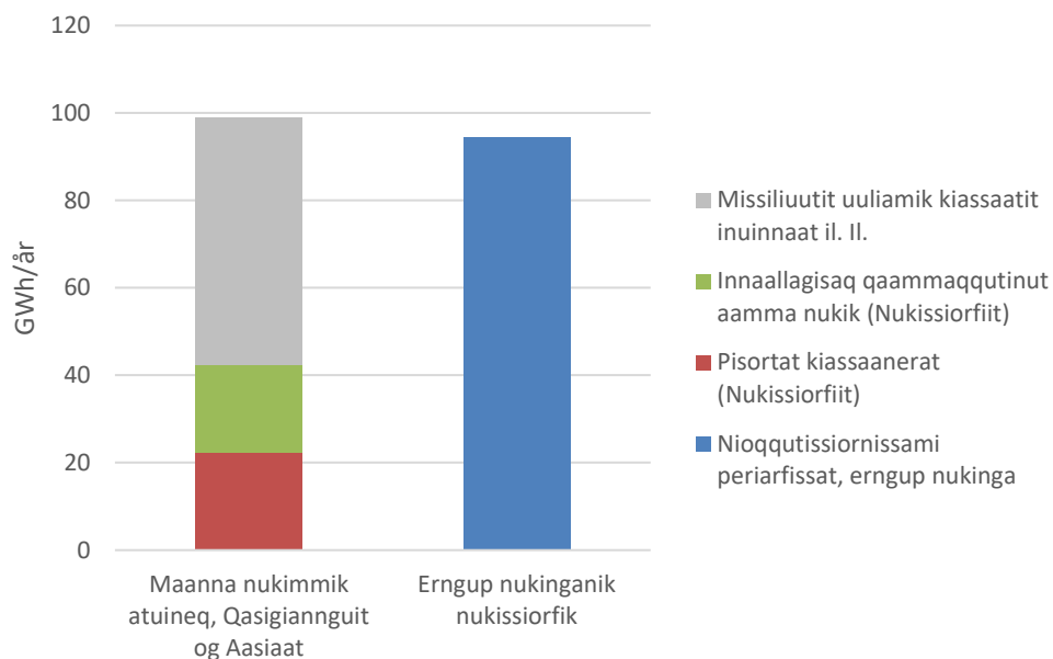
Figuri 2. Qasigianguani aamma Aasianni nukissiuutinik atuineq erngup nukinganik atuinermi periarfissamut sanilliullugu
