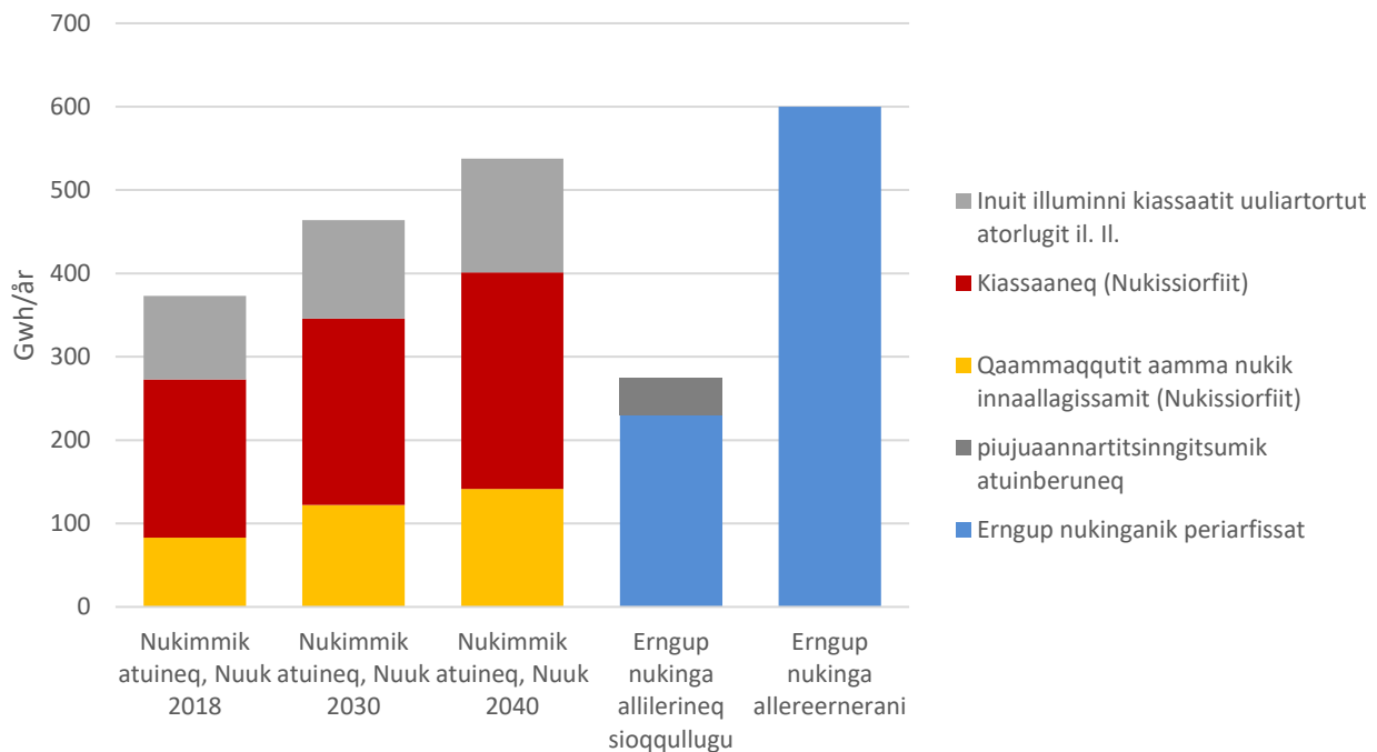
Figuri 7. Nuummi nukissiuutitik atuineq erngup nukinganik iluaquteqarnermit sanilliusilluni.
